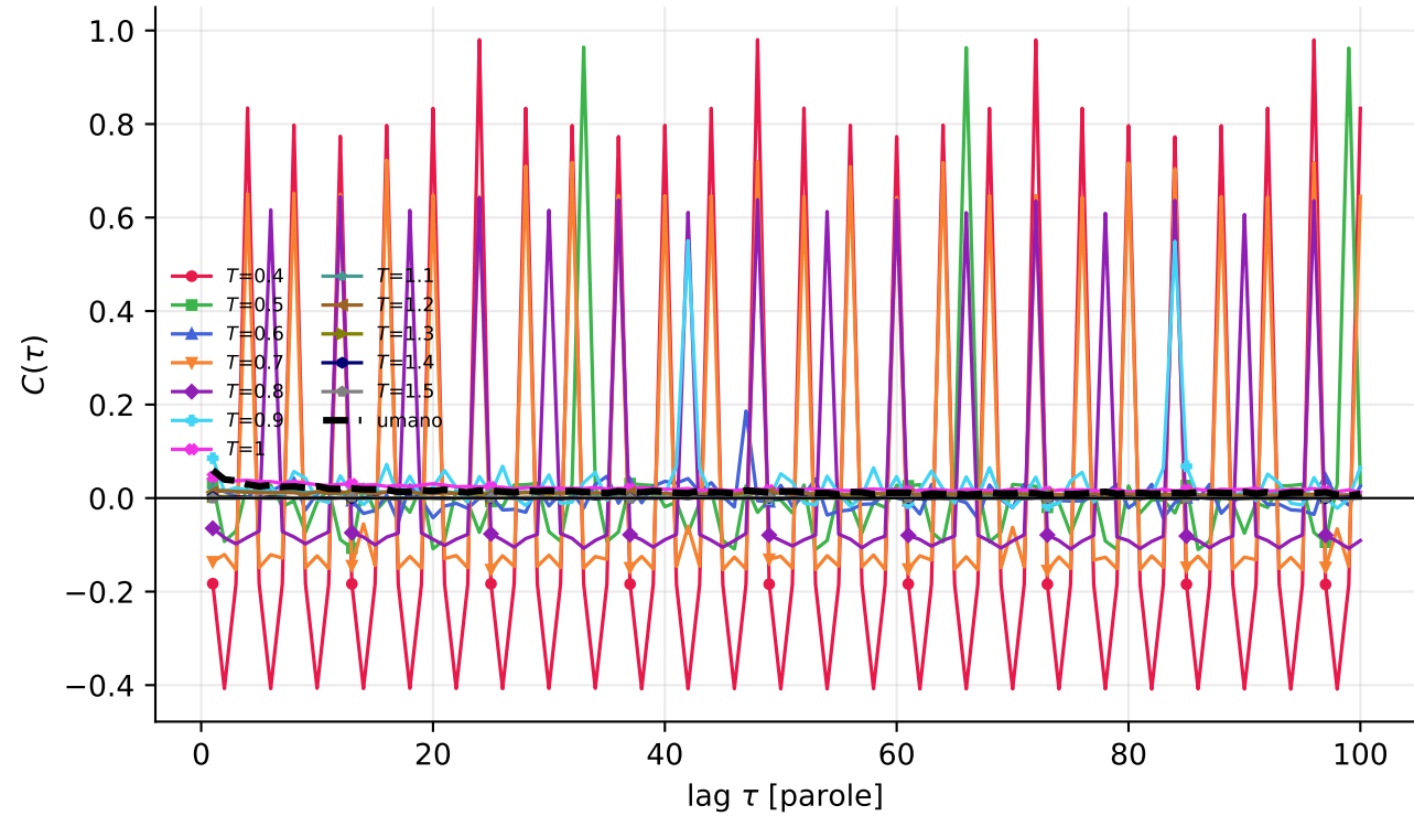
ACF a lag corti — Qwen2.5-14B (cfr. [F] Fig. 5-6)
